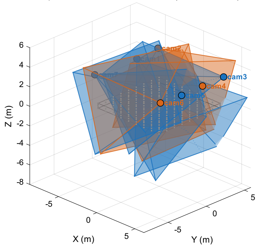
OptiTrack ad-hoc — 7 cams (Cost: 0.1449)
